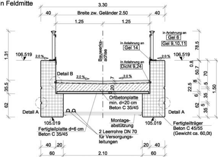
Querschnitt Überbau M 1:25
