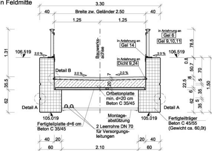
Querschnitt Überbau M 1:25 in Feldmitte
